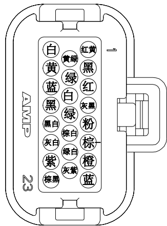
安普23P公胶壳(功能接口)
