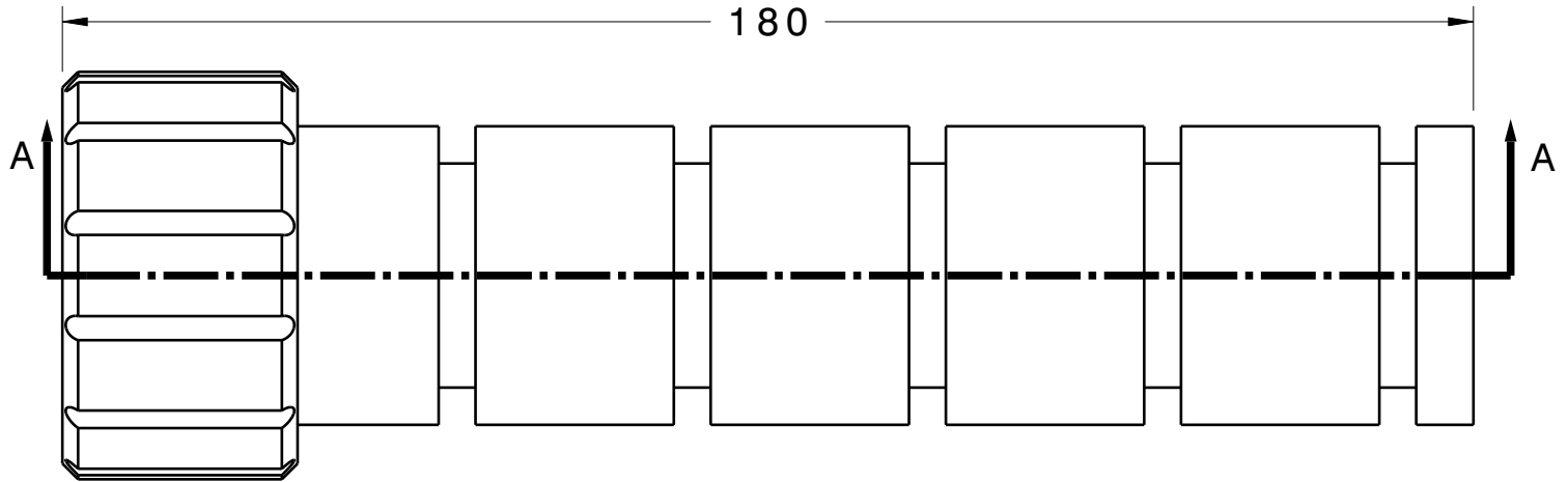
Right view Scale: 1:1
