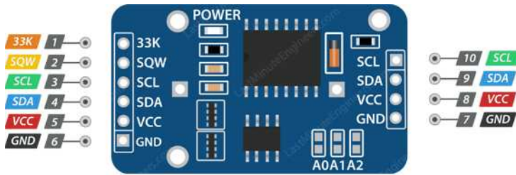
DS3231
