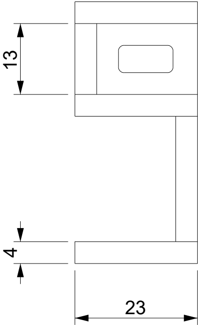
VISTA TRASERA
