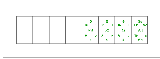
Template for 8 Dig x 7 Seg Display
