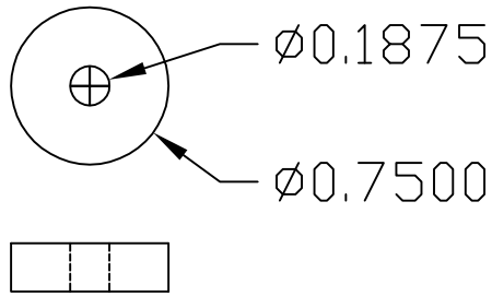
Motor Spacer (3)
