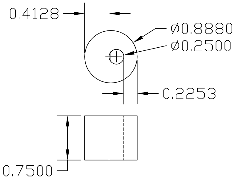
Cam (Oak)
