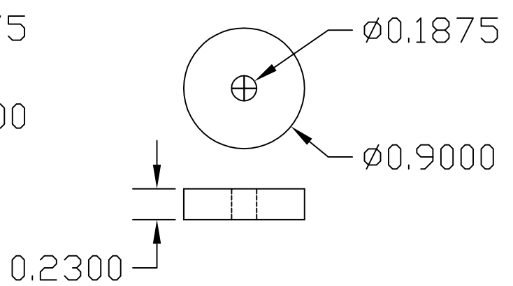
Arm Spacer
