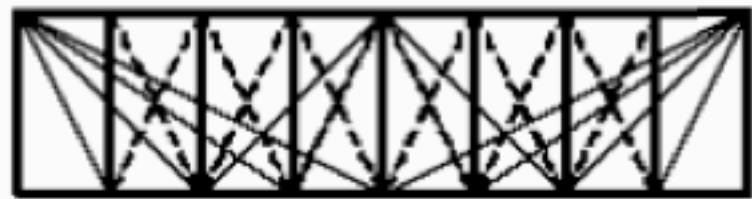
Fink
