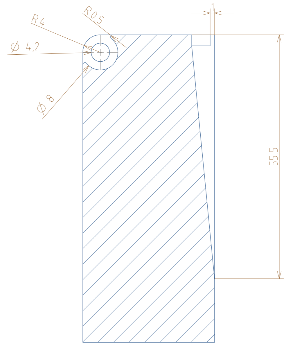
SECTION A-A
