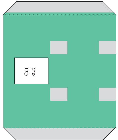
Box Top
