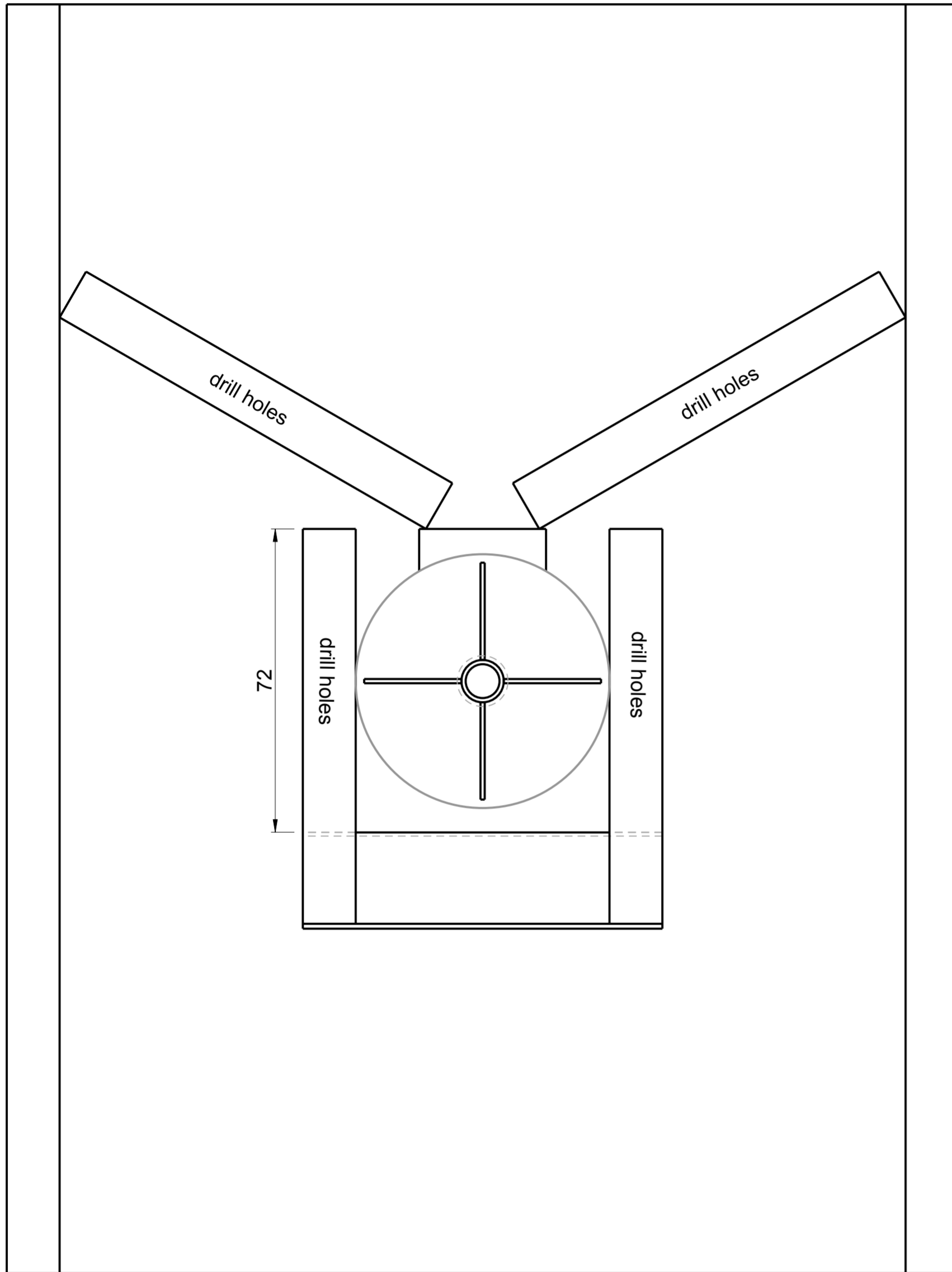
SECTION A-A
