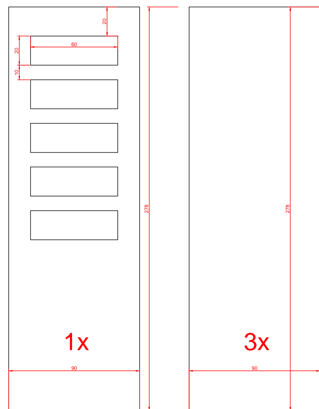
Wanden/deuren
