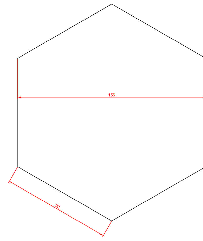
Vloerplaat
