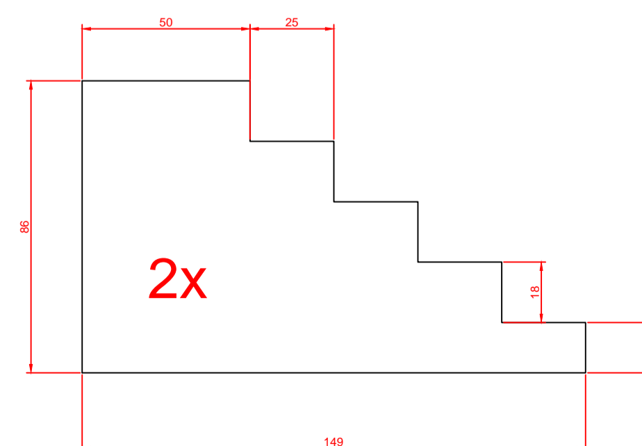
Traptreden
